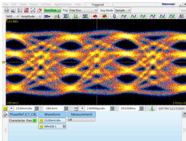
112 GBaud (224 Gbps) 135 mV Input Signal
